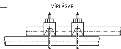
SAMTENGING STEYPUSTEINA SETJA SKAL TVO VÍRLÁSA Á HVER SAMSEYTI
