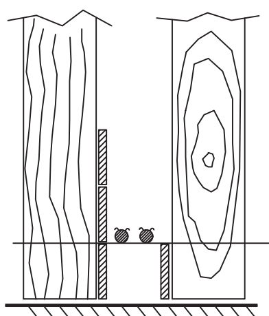
SNID A - A Í SÖKKULVEGG SÝND ERU 2 NEDSTU STEYPU- STYRKJARJÄRN Í STEYPUMÖTI OFAN Á NEDSTU MÖTAVÍRUM
